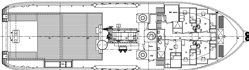
Maindeck
